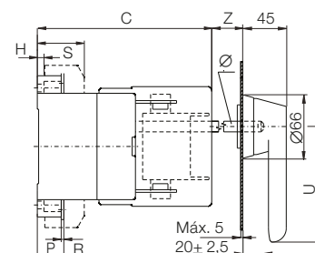
Versão com manopla montada na porta do painel
