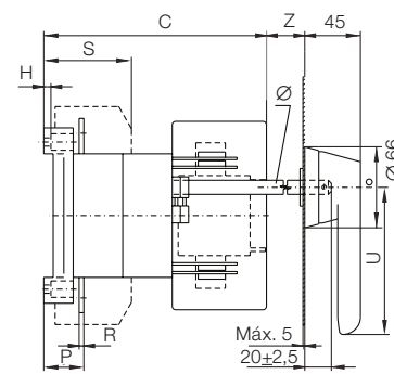
Versão com manopla montada na porta do painel
