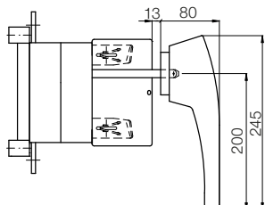
Versão com manopla interna montada sobre o eixo para RFW 630
