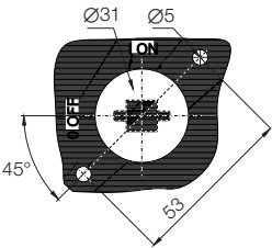
Furação para fixação da manopla
