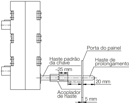
Montagem da haste de prolongação
