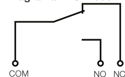
Diagrama - FSW 630
