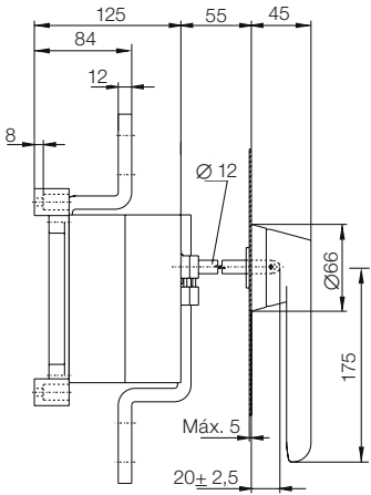
Versão com manopla montada na porta do painel
