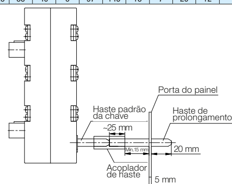
Montagem da haste de prolongação
